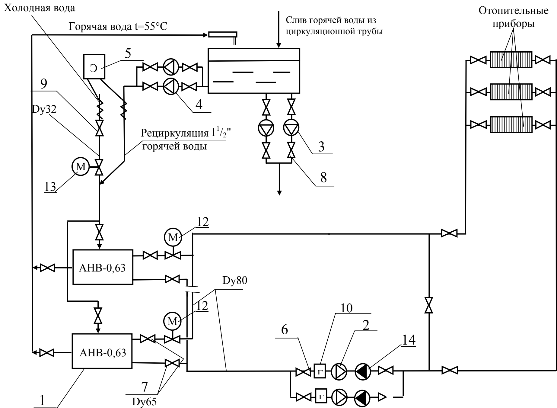
Автономная схема отопления общежития
